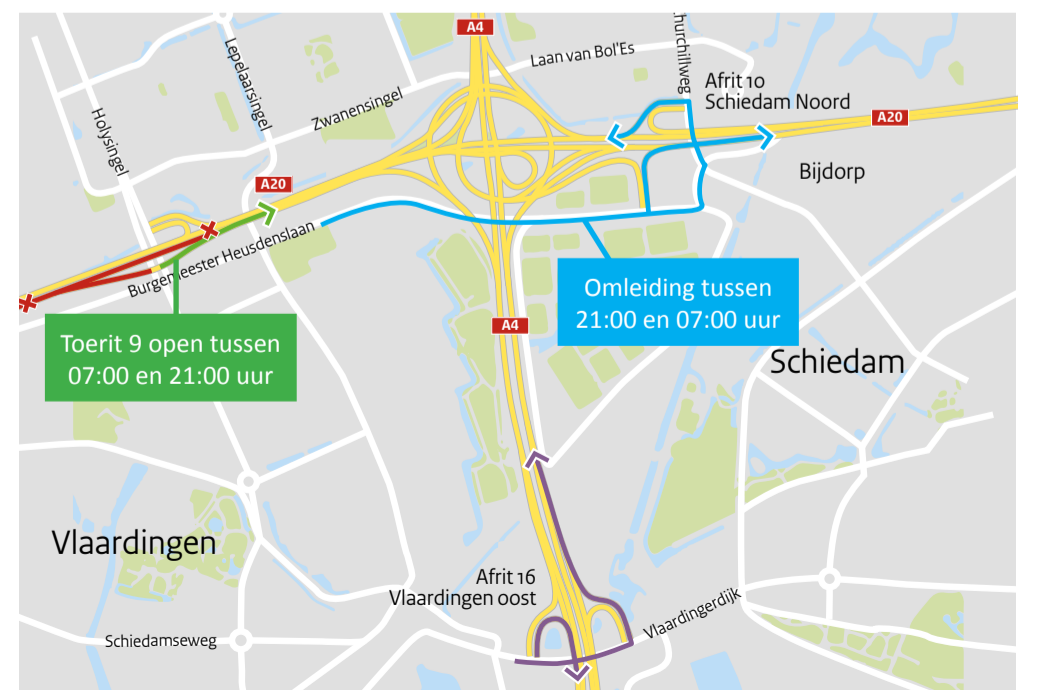
Afbeelding 8 Omleidingsroute lokaal verkeer Vlaardingen naar A20 richting Rotterdam
