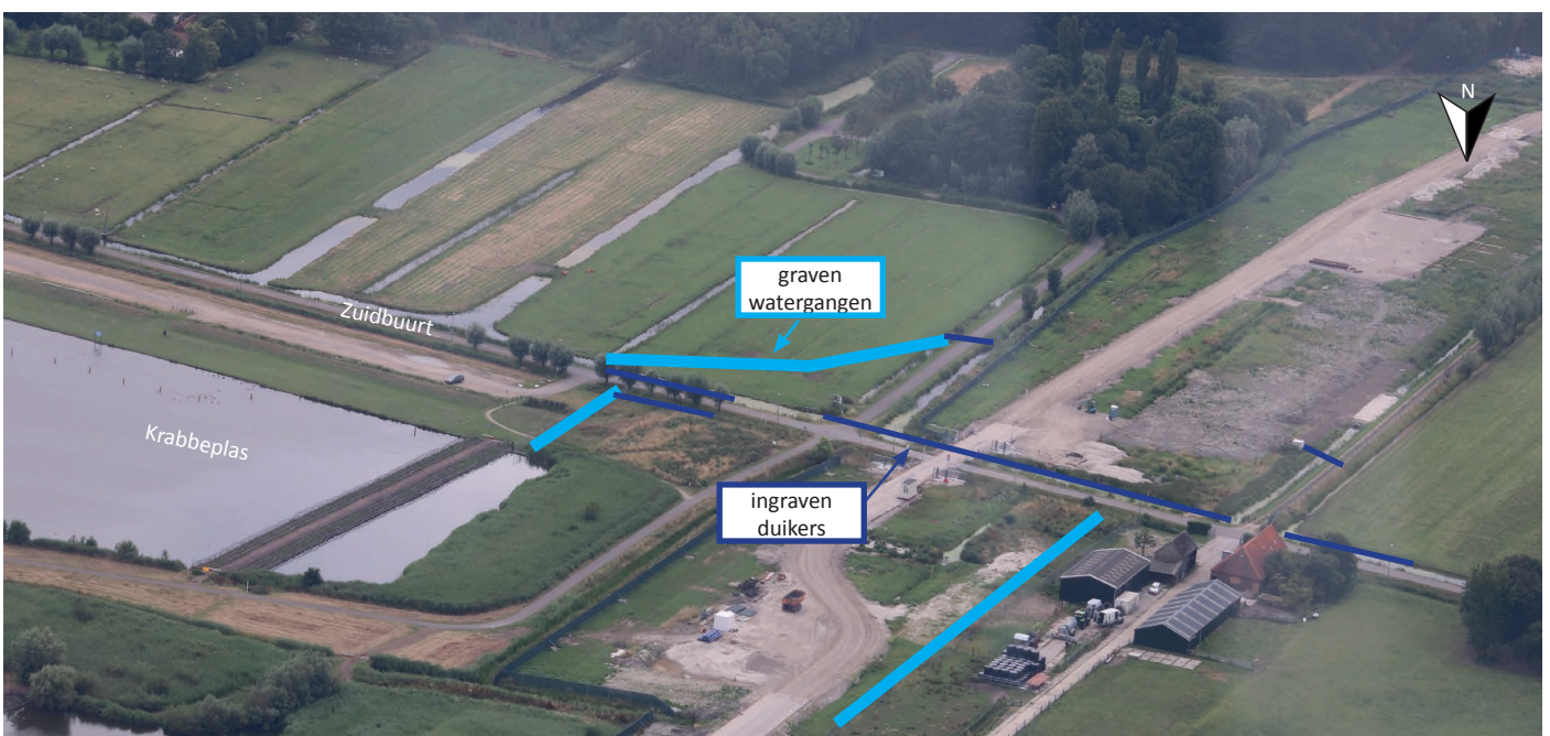
Afbeelding 2 Locaties aanbrengen watergangen en duikers
