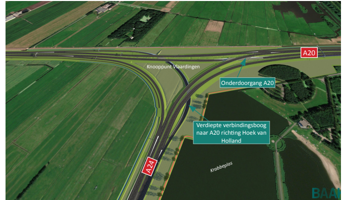
Afbeelding 1 Ontwerp knooppunt Vlaardingen
