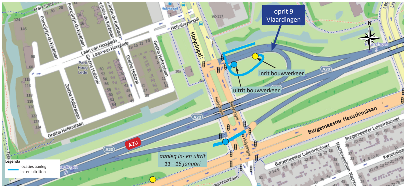
Afbeelding 1 Locaties in- en uitrit werkverkeer bij A20 oprit 9 Vlaardingen 25-29 januari
