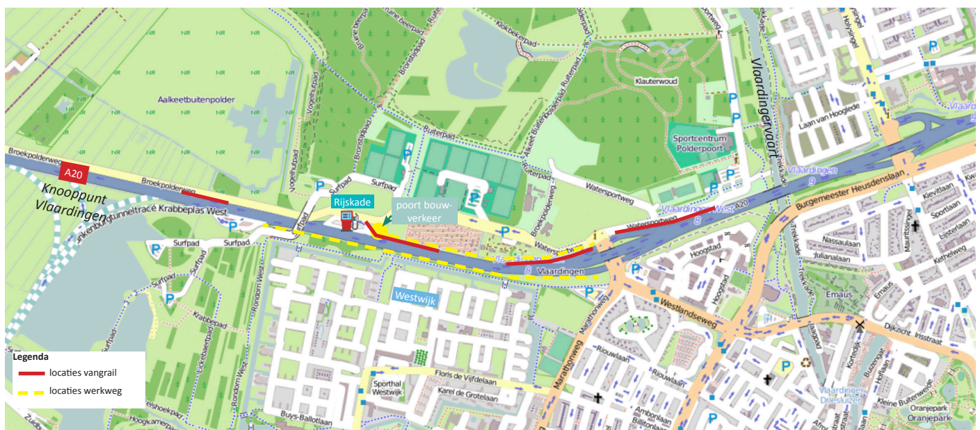
Afbeelding 1 Locatie plaatsen vangrail en bouwwegen
